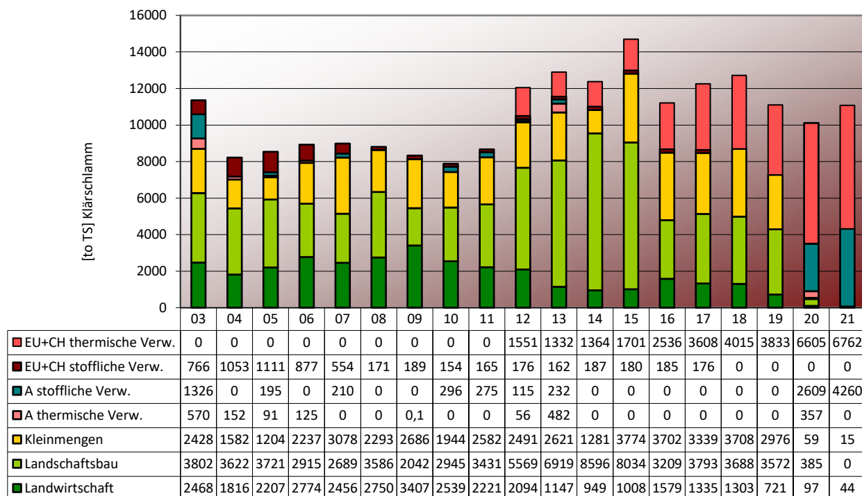
Abbildung 7: Verwertungsarten in Vorarlberg 2003-2021 (Mengen in to TS)
